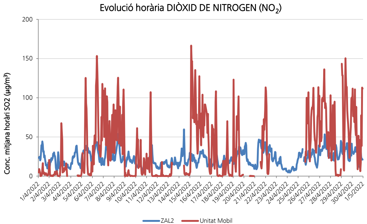
Figura 7: Evolució horària del NO 2 .
