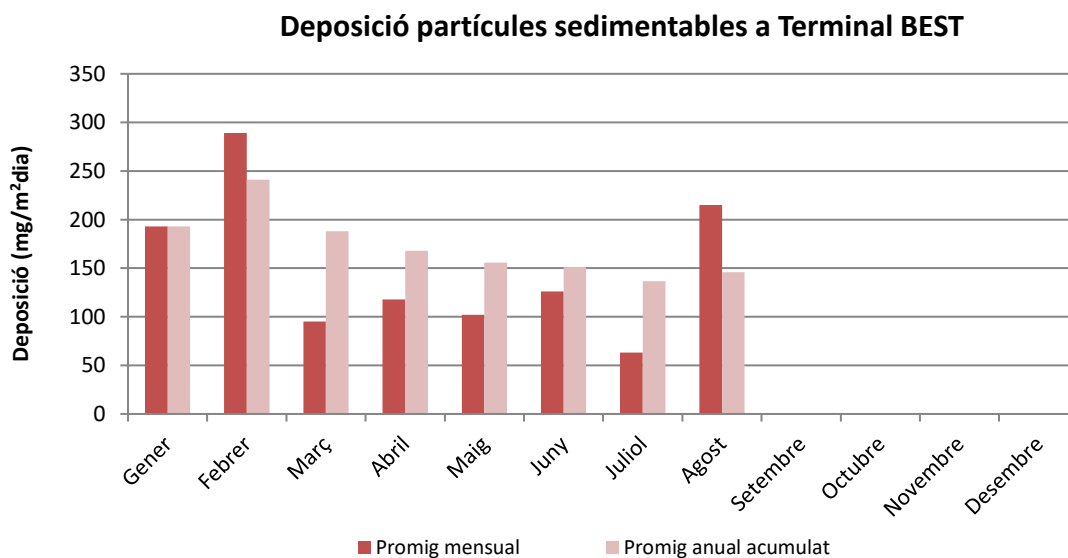
Figura 5: Gràfic anual d'evolució mensual de la deposició de partícules sedimentables
