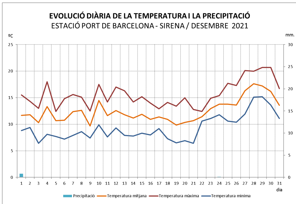
Figura 8: Evolució de la temperatura i la precipitació durant el mes de desembre a l'estació Sirena.
