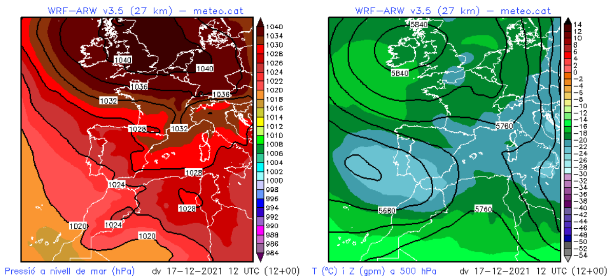
Figura 4: Mapa de pressió en superfície (esquerra) i a 500 hPa (dreta) del dia 17 de desembre a les 12:00 hores UTC. Es va assolir el màxim de pressió atmosfèrica amb 1031,6 hPa a Dispensari.
