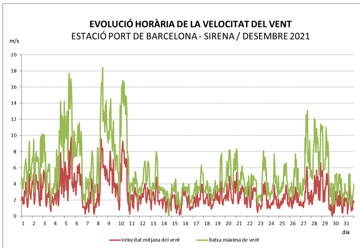
Figura 9: Evolució del vent durant el mes de desembre a l'estació Sirena.
