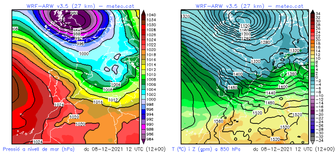
Figura 3: Mapa de pressió en superfície (esquerra) i a 850 hPa (dreta) del dia 8 de desembre a les 12:00 hores UTC. Va ser la jornada més ventosa, amb una ratxa màxima de 73 km/h a Adossat.
