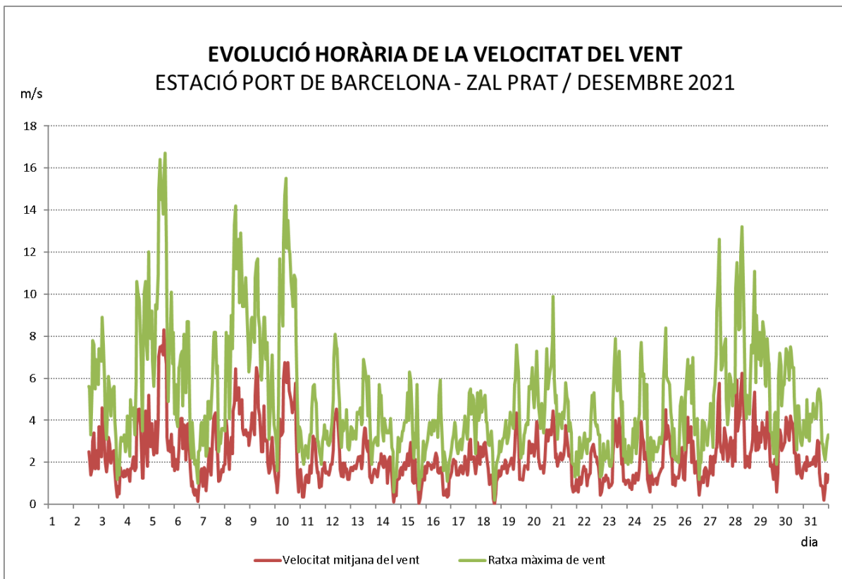
Figura 6: Evolució del vent durant el mes de desembre a l'estació Port de Barcelona - ZAL Prat.
