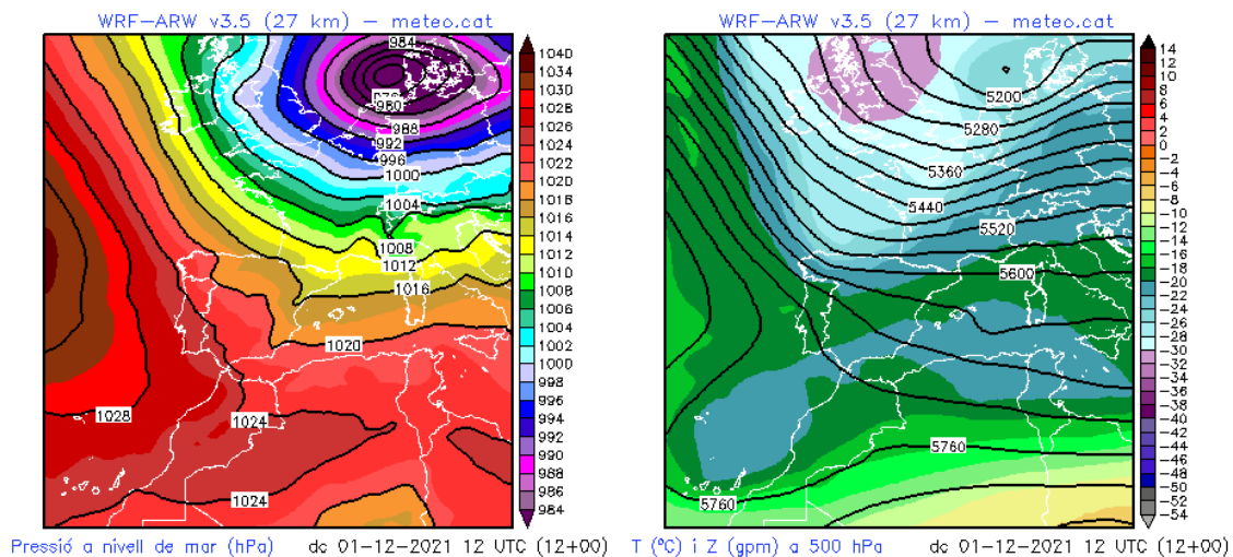
Figura 2: Mapa de pressió en superfície (esquerra) i a 500 hPa (dreta) del dia 1 de desembre a les 12:00 hores UTC. L'inici de mes va precipitar de forma minsa a la zona portuària, sent al final l'episodi més destacat.
