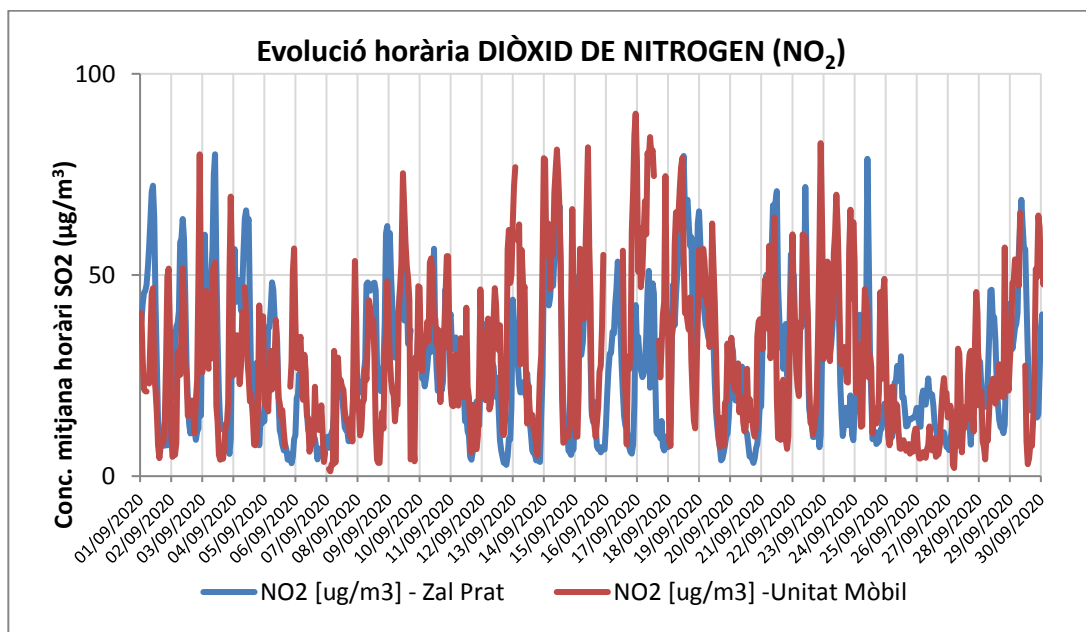
Figura 7: Evolució horària pel mes de setembre del NO 2 als punts de mesura del Port de Barcelona.
