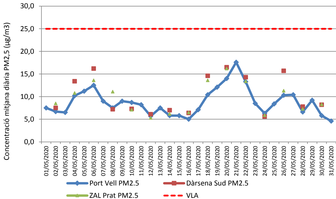
Figura 4: Gràfic d'evolució diària durant el mes de maig dels valors de PM 2,5 i el valor de referència VLA.
