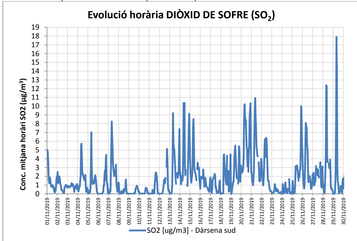
Figura 6: Evolució horària del SO 2 a Dàrsena sud i Unitat mòbil.
