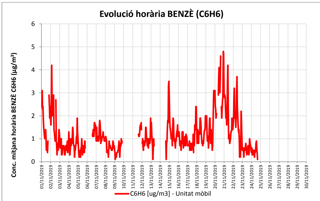
Figura 7: Evolució horària pel mes de novembre del C 6 H 6 a la Unitat mòbil.
