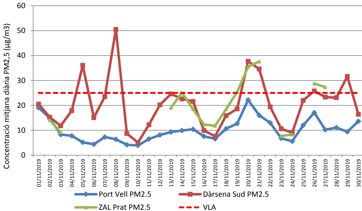
Figura 4: Gràfic d'evolució diària durant el mes de novembre dels valors de PM 2,5 i el valor de referència VLA.
