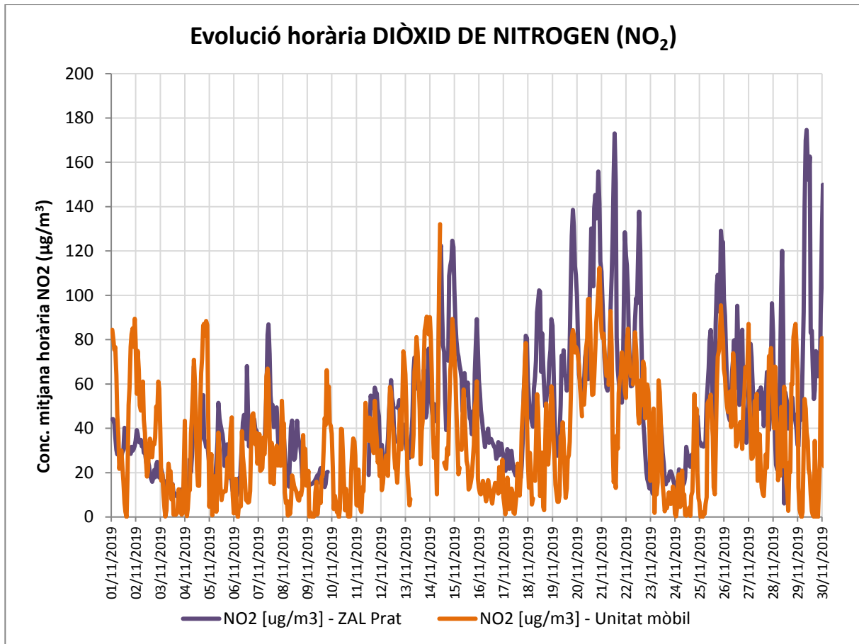
Figura 7: Evolució horària pel mes de novembre del NO 2 als punts de mesura del Port de Barcelona.
