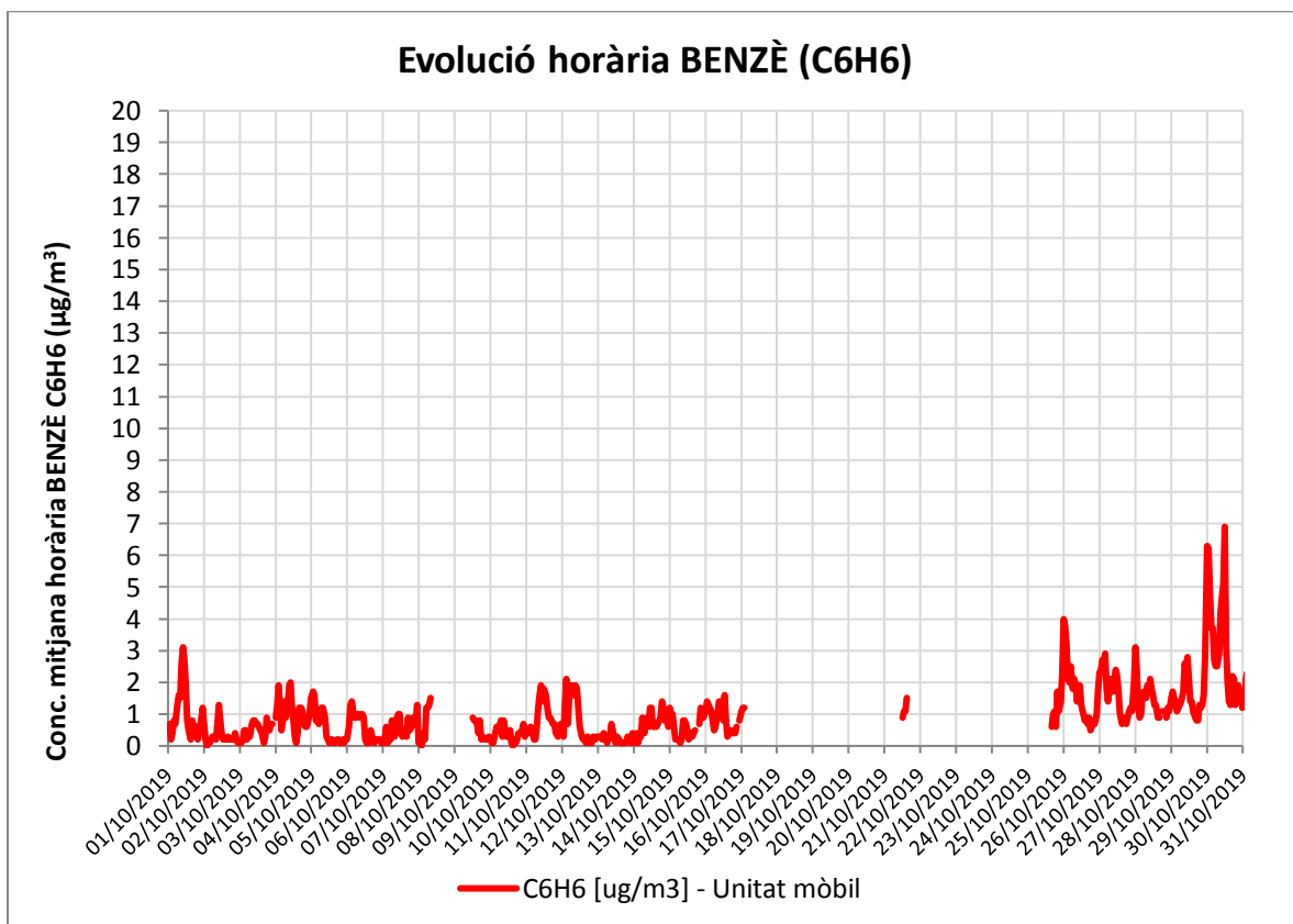
Figura 7: Evolució horària pel mes d'octubre del C 6 H 6 a la Unitat mòbil.
