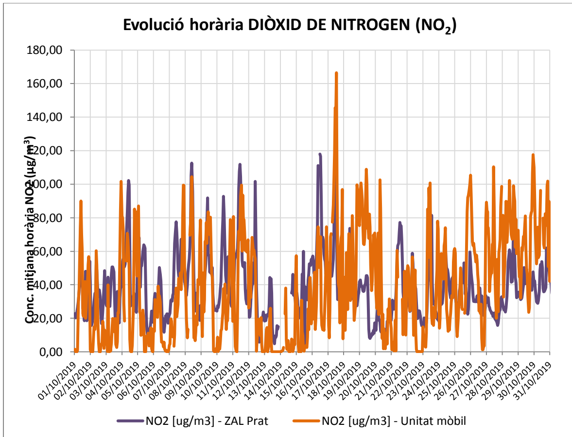
Figura 7: Evolució horària pel mes d'octubre del NO 2 als punts de mesura del Port de Barcelona.
