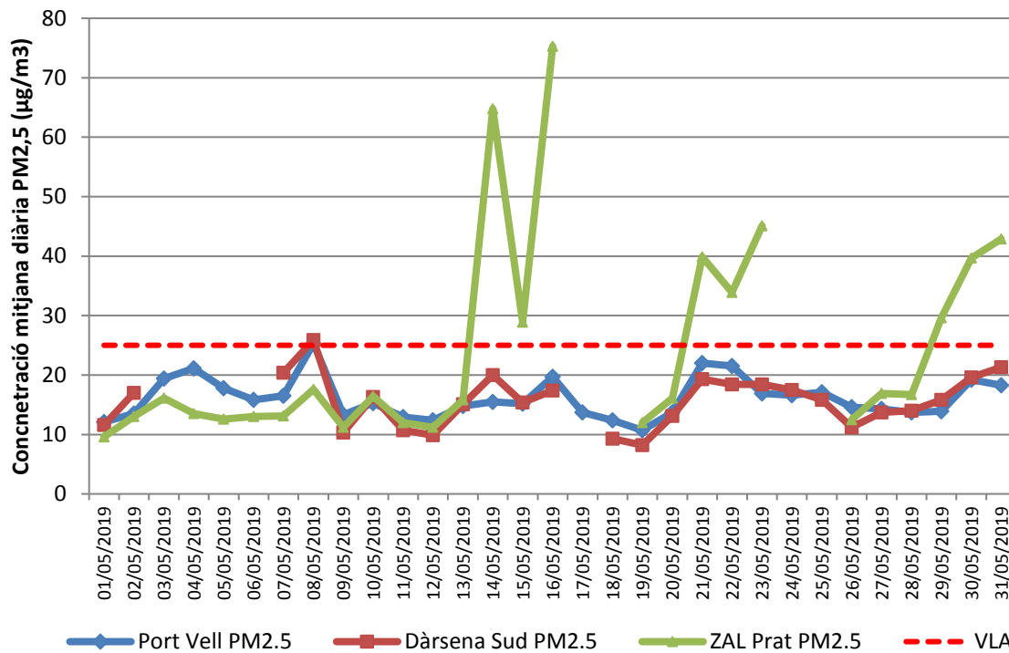
Figura 4: Gràfic d'evolució diària durant el mes de maig dels valors de PM 2,5 i el valor de referència VLA.
