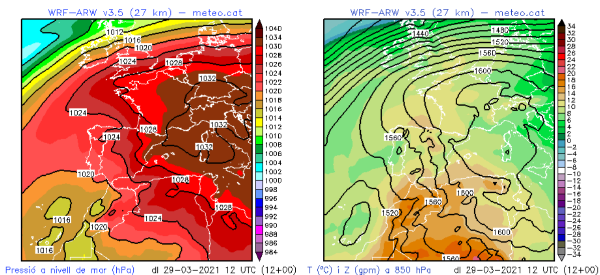
Figura 4: Mapa de pressió en superfície (esquerra) i a 850 hPa (dreta) del dia 29 de març a les 12:00 hores UTC. L'anticicló entre els dies 29 i 31 de març va facilitar l'arribada de masses d'aire càlid tropical amb entrada de pols sahariana. Es va registrar un màxim de pressió atmosfèrica de 1031.6 hPa a l'estació portuària Dispensari.
