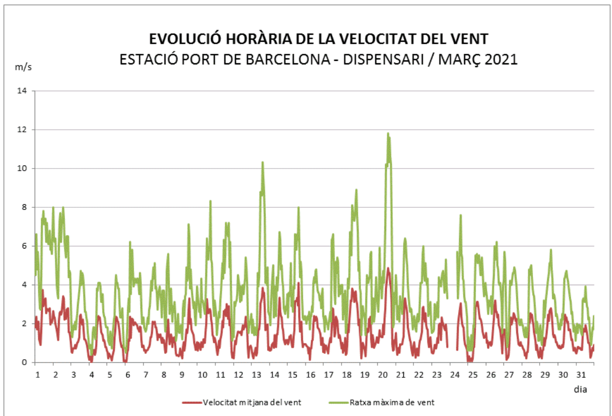
Figura 12: Evolució del vent durant el mes de març a l'estació Dispensari.
