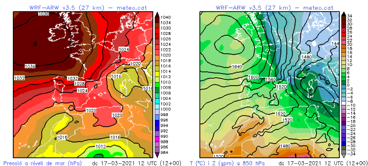
Figura 2: Mapa de pressió en superfície (esquerra) i a 850 hPa (dreta) del dia 17 de març a les 12:00 hores UTC. El mes de març ha estat càlid, registrant una temperatura màxima mensual de 20.2 °C el dia 17 a l'estació Dispensari.
