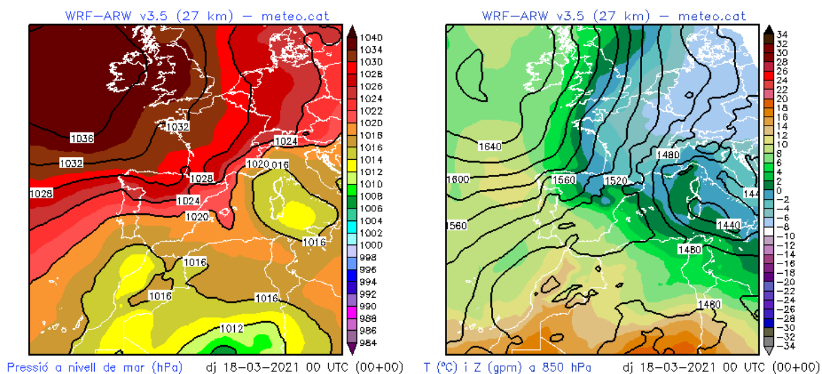
Figura 3: Mapa de pressió en superfície (esquerra) i a 850 hPa (dreta) del dia 18 de març a les 00:00 hores UTC. L'episodi de vent i fred entre els dies 17 i 21 va produir precipitació que va acumular un total de 6.1 mm a l'estació portuària Dispensari, en un mes que ha estat sec.
