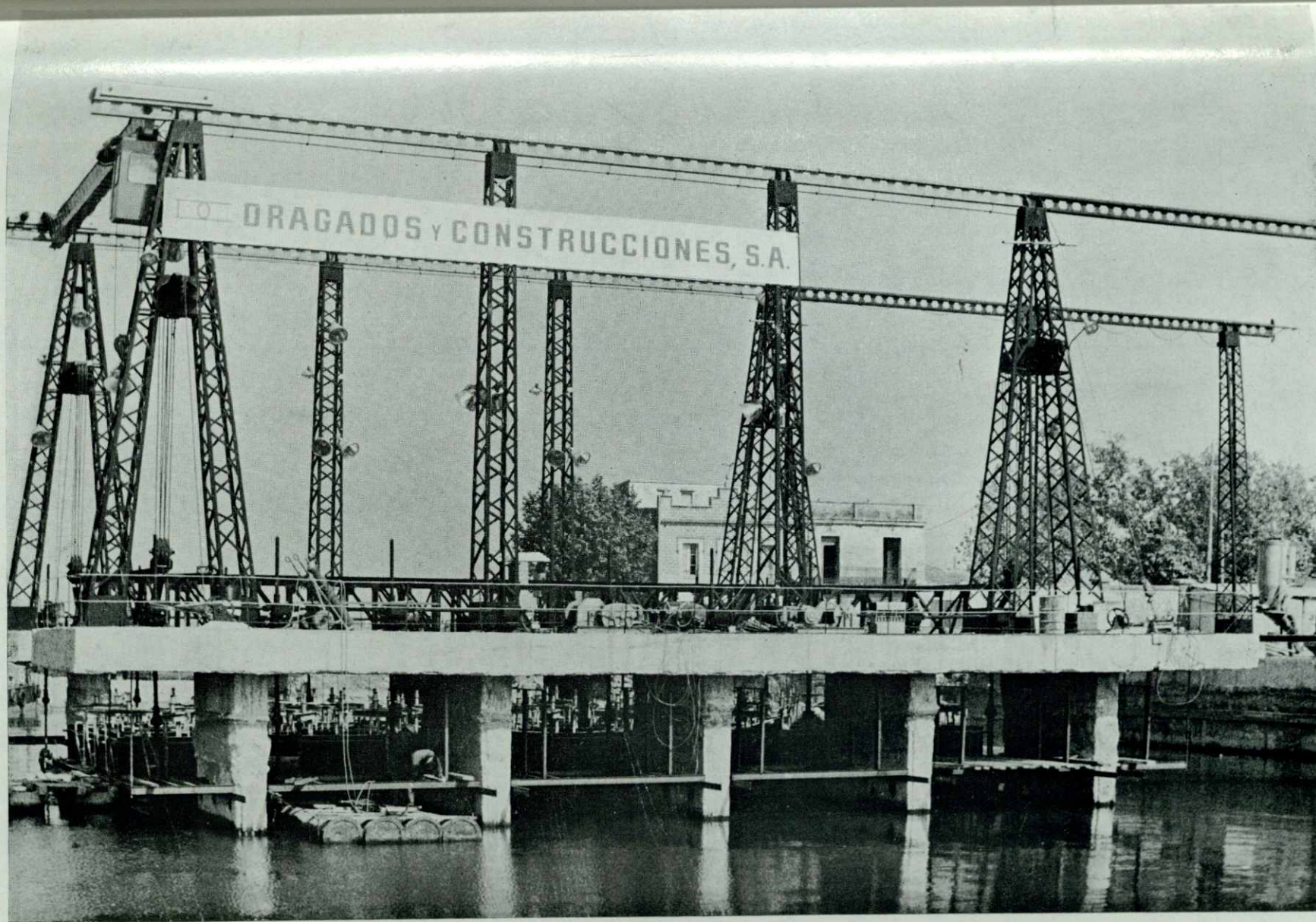
Instalación para la construcción de los cajones flotantes de hormigón, armado para el muelle de Containers
