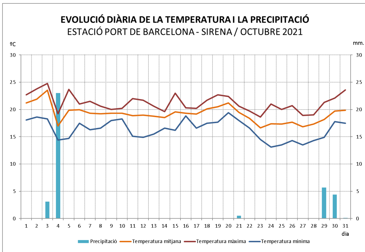
Figura 8: Evolució de la temperatura i la precipitació durant el mes d'octubre a l'estació Sirena.
