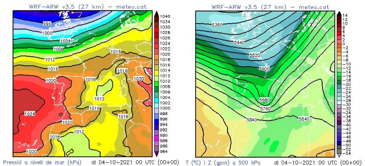
Figura 2: Mapa de pressió en superfície (esquerra) i a 500 hPa (dreta) entre el dia 3 i el 4 d'octubre. Va ser el primer dels dos episodis de l'octubre pel que fa precipitació. L'estació portuària Dispensari va acumular 30 mm entre els dos dies.
