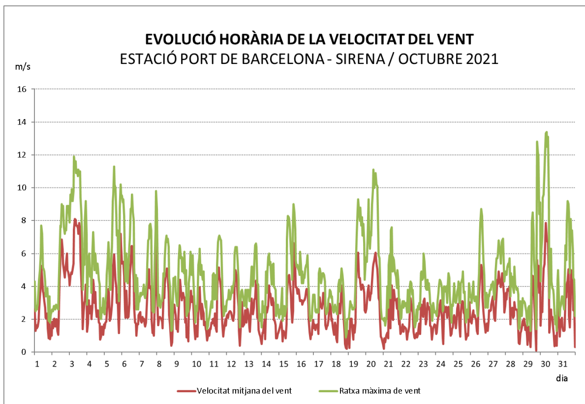
Figura 9: Evolució del vent durant el mes d'octubre a l'estació Sirena.
