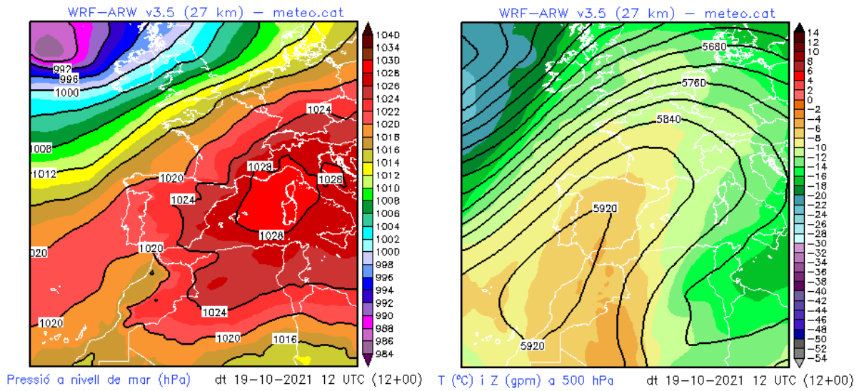
Figura 3: Mapa de pressió en superfície (esquerra) i a 500 hPa (dreta) del dia 19 d'octubre a les 12:00 hores UTC. La pressió atmosfèrica màxima es va assolir a l'estació portuària Dispensari on es van registrar 1027.1 hPa.
