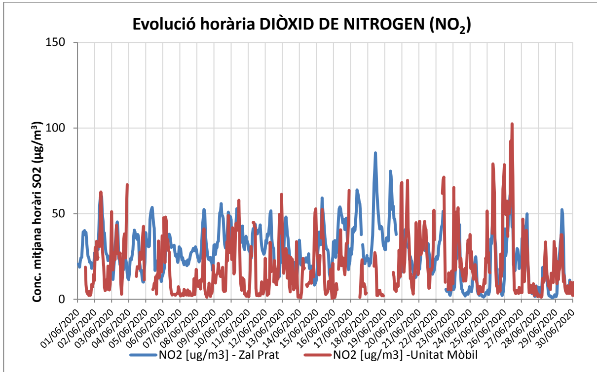
Figura 7: Evolució horària pel mes de juny del NO 2 als punts de mesura del Port de Barcelona.
