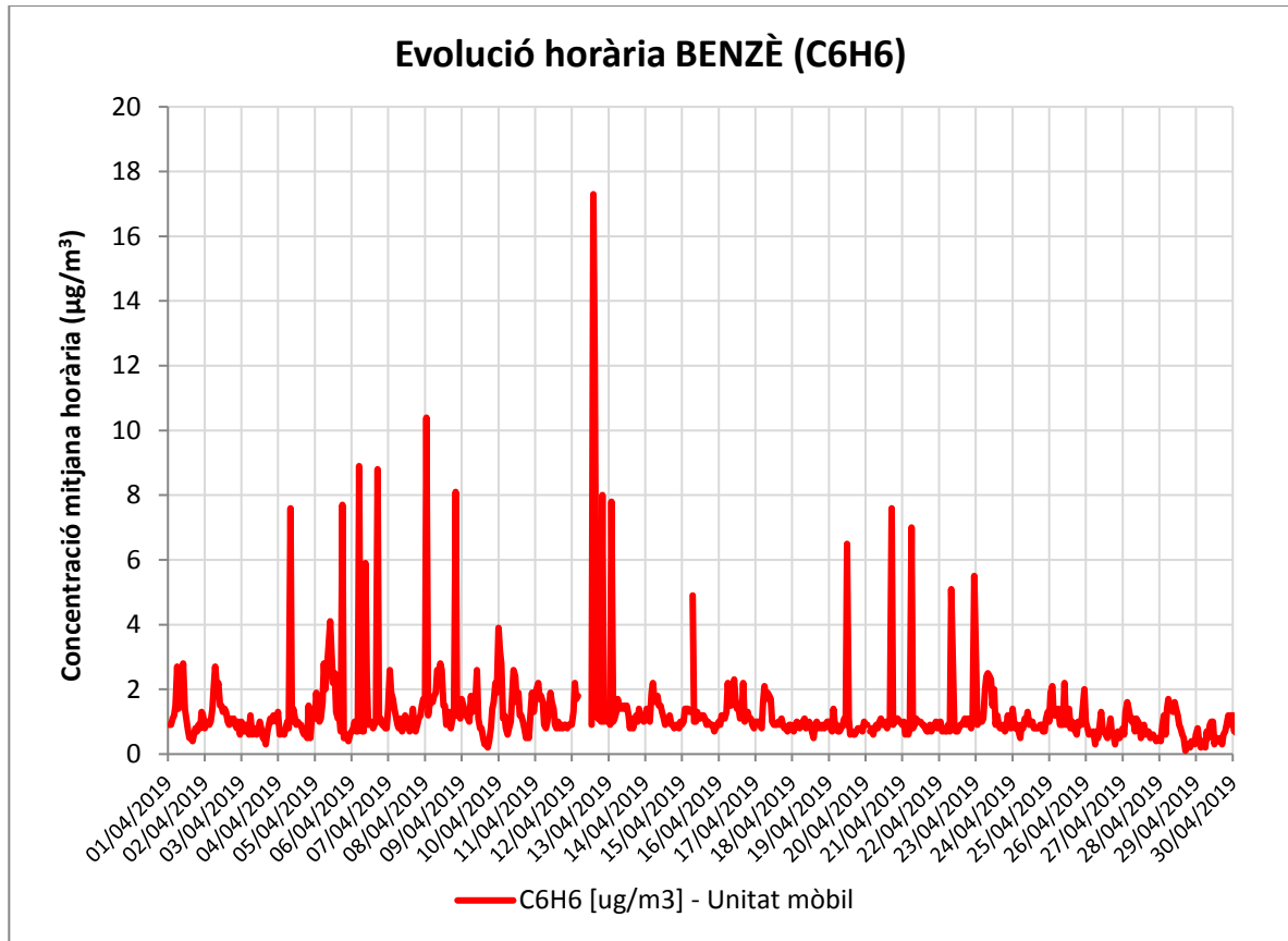
Figura 7: Evolució horària pel mes d'abril del C6H6 a la Unitat mòbil.
